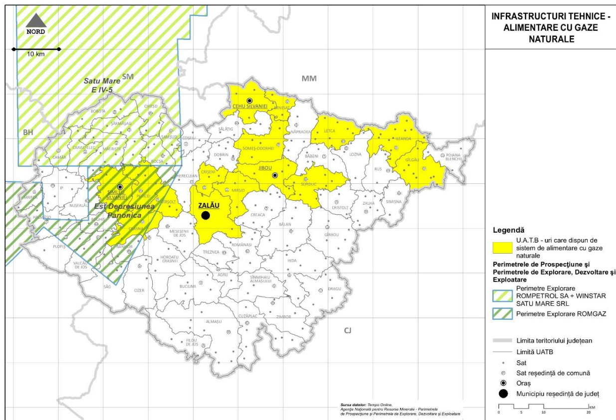
Figura 31: Alimentare cu gaze naturale
